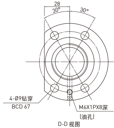
D-D 视图
