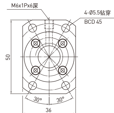
D-D 视图
