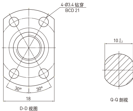
D-D 视图
