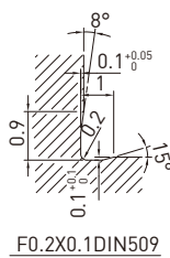
X 详图
