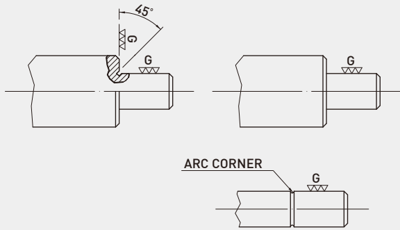
图A.2 滚珠丝杠肩部的设计
