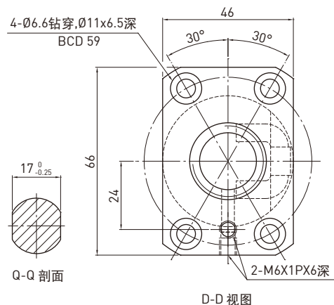
D-D 视图
