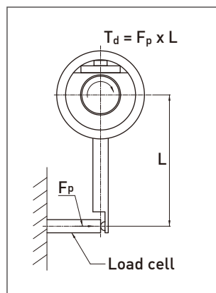
图 4.20 预压扭力量测方法(同 JIS B1192)
