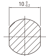
Q-Q 剖视
