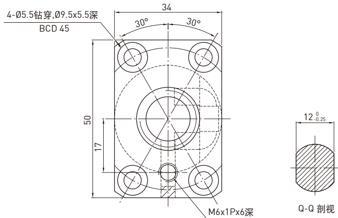
D-D 视图
