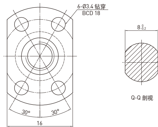
D-D 视图
